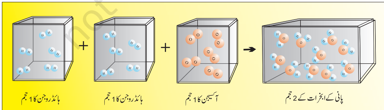
شکل 1.9 ہائڈروجن کے 2 حجم، آکسیجن کے 1 حجم سے تعامل کر کے پانی کے ابخراات کے 2 حجم دیتے ہیں
