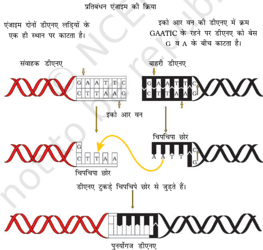
चित्र 11.1 प्रतिबंधन एंजाइम - इको आर वन (EcoRI) की क्रिया द्वारा पुनर्योगज डीएनए के निर्माण के चरण
