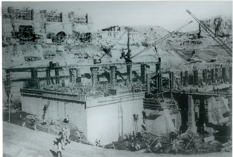
شکل 7 - گاندھی ساگر باندھ پر کام جاری ہے یہ ان چار میں سے پہلا باندھ ہے جو مدھیہ پردیش میں چمبل دریا پر بنائے گئے۔ 1960 میں مکمل ہوا تھا۔
