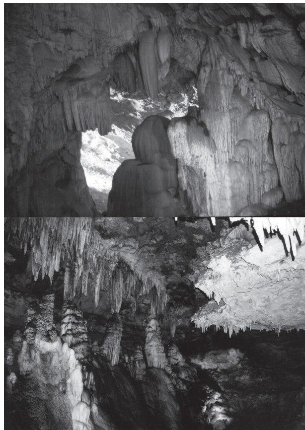
चित्र 7.10 : चूना पत्थर गुफा में स्टैलेक्टाइट एवं स्टैलेग्माइट
