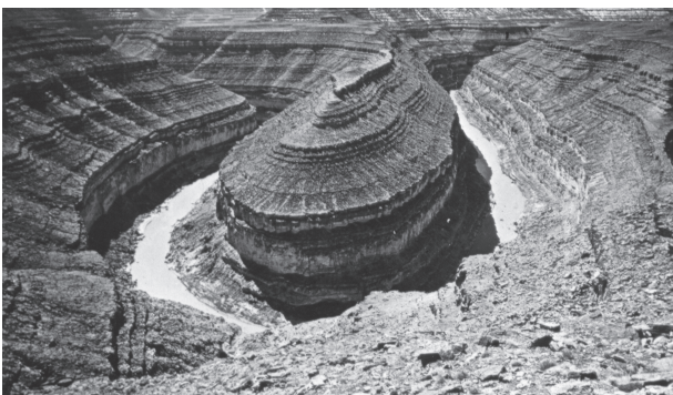
चित्र 7.2 : संयुक्त राज्य अमेरिका में कोलोरेडो का गभीरीभूत विसर्प लूप, जो इसकी घाटी के कैनियन जैसे सोपान सदृश्य पार्श्वीय ढाल दर्शाता है।
