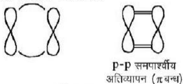
चित्र 8.6 : \pi बन्ध
