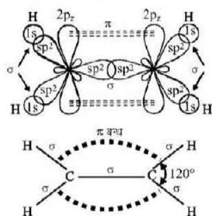
चित्र 8.9 : एथीन की कक्षकीय संरचना
