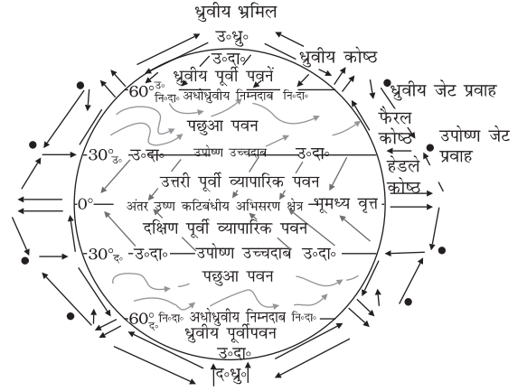
चित्र 10.6 : वायुमंडल का सरलतम सामान्य परिसंचरण
