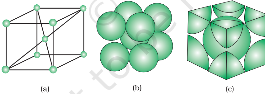
شکل 1.14: ایک جسم مرکزی مکعبی یونٹ سیل (a) کھلی ساخت (b) جگہ پُر کرنے والی ساخت
