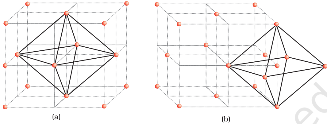
شکل 2: CCP یا شکل FCC جالی کے ایک یونٹ سیل ہشت پہلو خلاؤں کا وقوع (a) مکعب کے جسمی مرکز (Body Centre) اور (b) ہر کنارے کے مرکز پر (یہاں صرف ایک خلا دکھایا گیا ہے)
