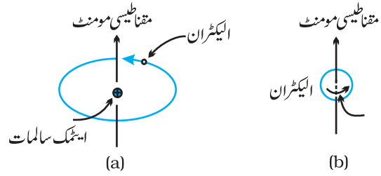
شکل 1.35: اس مقناطیسی معیاری اثر کا اظہار جو وابستہ ہے (a) کسی آرٹھنگ الیکٹرون سے اور (b) گردشی الیکٹرون سے
