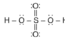
\text{H}_2\text{SO}_4
