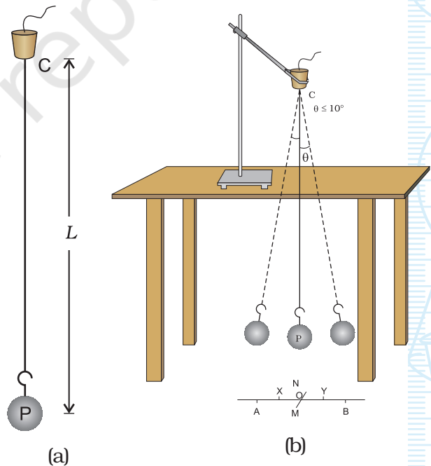
चित्र 40.2: (a) विभक्त कॉर्क में दृढ़ सरल लोलक तथा (b) सरल लोलक की लम्बाई में परिवर्तन के साथ उसके आवर्त काल में परिवर्तन के अध्ययन के लिए प्रयोगिक व्यवस्था।
