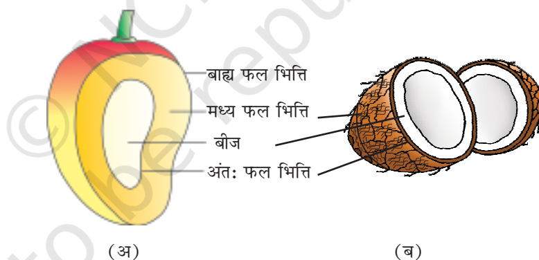
चित्र 5.17 फल के भाग (अ) आम (ब) नारियल
