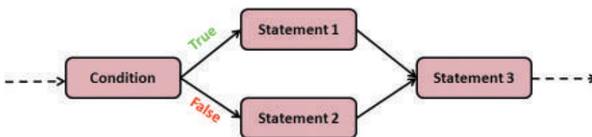
Fig. 3.9 : Selection structure
