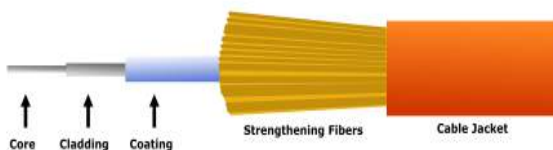
Fig. 8.5 : Optical Fibre
