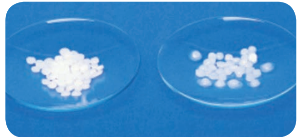
படம் 9.11 ஈரம் உறிஞ்சிக் கரையும் சோடியம் ஹைட்ராக்சைடு.
