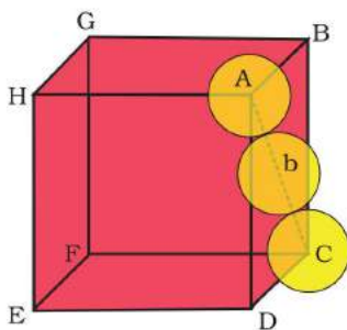
चित्र 1.24—घनीय निविड संकुलित संरचना स्पष्ट करने हेतु दूसरे कोनों में गोलकों को नहीं रखा गया है।
