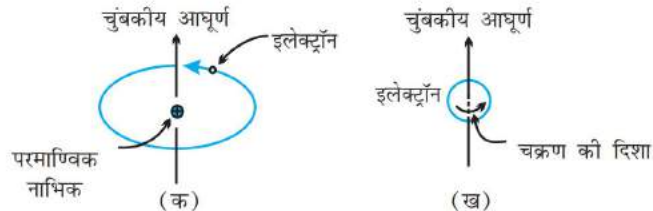
चित्र 1.35—(क) इलेक्ट्रॉन की कक्षीय गति, (ख) इलेक्ट्रॉन की चक्रण गति के साथ संयुक्त चुंबकीय आघूर्ण का निदर्शन
