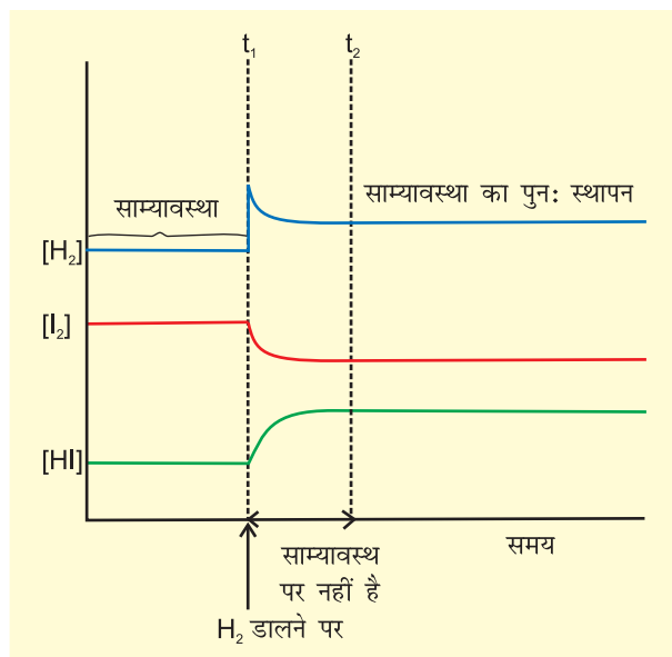
चित्र 7.8 \text{H}_2(\text{g}) + \text{I}_2(\text{g}) \rightleftharpoons 2\text{HI}(\text{g}) अभिक्रिया में साम्यावस्था पर \text{H}_2 के डालने पर अभिकारकों एवं उत्पादों के सांद्रण में परिवर्तन
