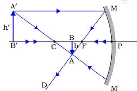
चित्र 38.1 : अवतल दर्पण MM' (जिसकी फोकस दूरी f तथा वक्रता त्रिज्या R है) द्वारा प्रतिबिम्ब A'B' बनना जबकि बिम्ब AB दर्पण के वक्रता केन्द्र C तथा फोकस बिन्दु F के बीच स्थित है: एक वास्तविक, उल्टा तथा बड़े साइज का प्रतिबिम्ब A'B' दर्पण के वक्रता केन्द्र से दूर स्थित होता है।
