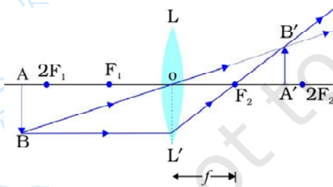
चित्र 45.1 : पतले उत्तल लेंस LL' द्वारा (जिसकी फोकस दूरी f है) 2f से थोड़ा अधिक दूरी पर रखे बिम्ब AB के प्रतिबिम्ब A'B' का बनना: एक वास्तविक, उल्टा तथा छोटा प्रतिबिम्ब A'B' , F_2 तथा 2F_2 के बीच में स्थित है। F_2 उत्तल लेंस का दूसरा मुख्य फोकस है।
