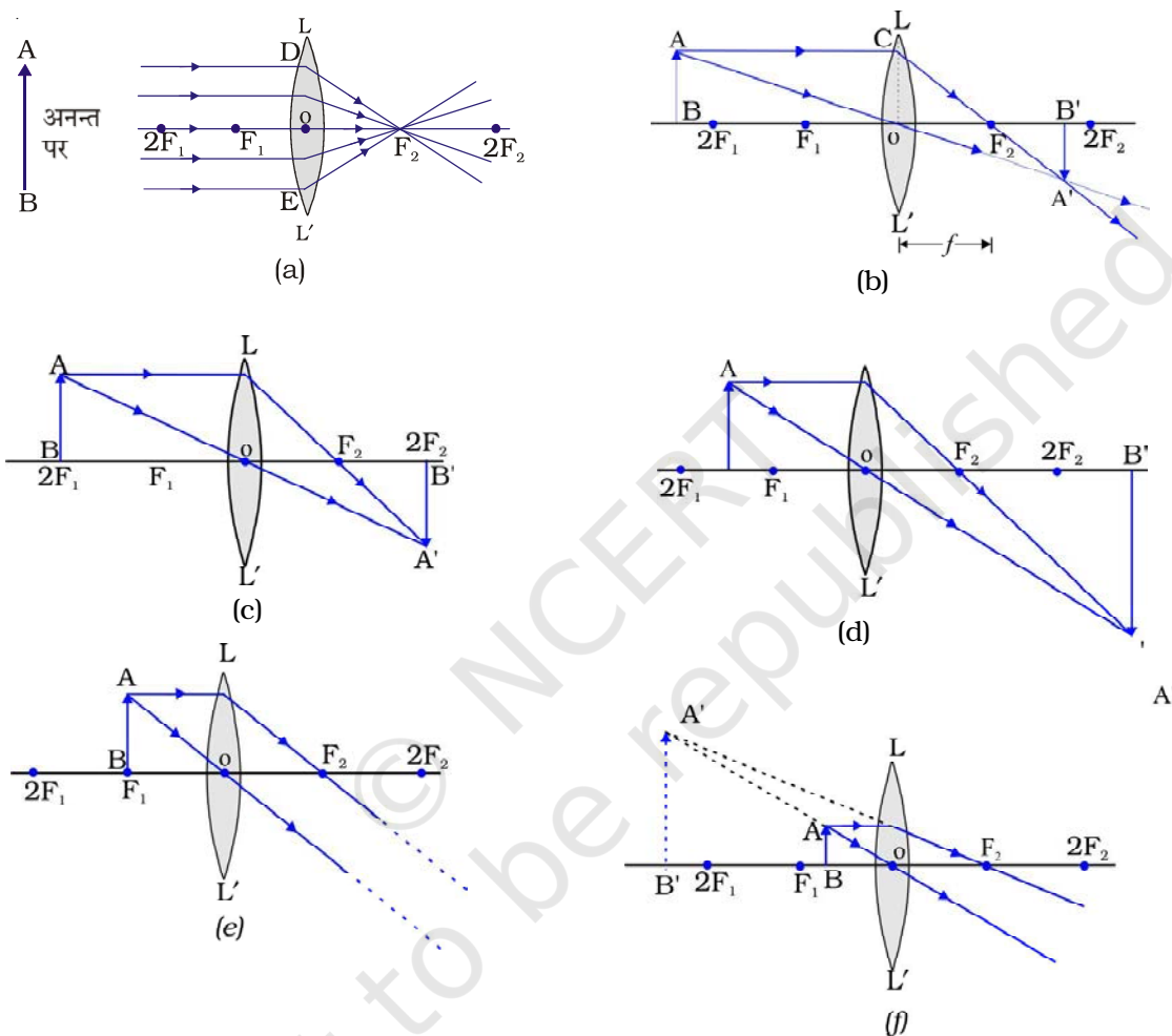
चित्र 43.4 : बिम्ब की विभिन्न स्थितियों के लिए उत्तल लेंस द्वारा बने प्रतिबिम्ब की स्थितियाँ, साइज एवं प्रकृति
