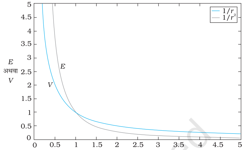
चित्र 2.4 किसी बिंदु आवेश Q के लिए दूरी r में परिवर्तन के साथ विभव में परिवर्तन ( Q/4\pi\epsilon_0 ) \text{m}^{-1} के मात्रकों में (नीला वक्र) तथा दूरी r में परिवर्तन के साथ विद्युत क्षेत्र में परिवर्तन ( Q/4\pi\epsilon_0 ) \text{m}^{-2} काला वक्र।
