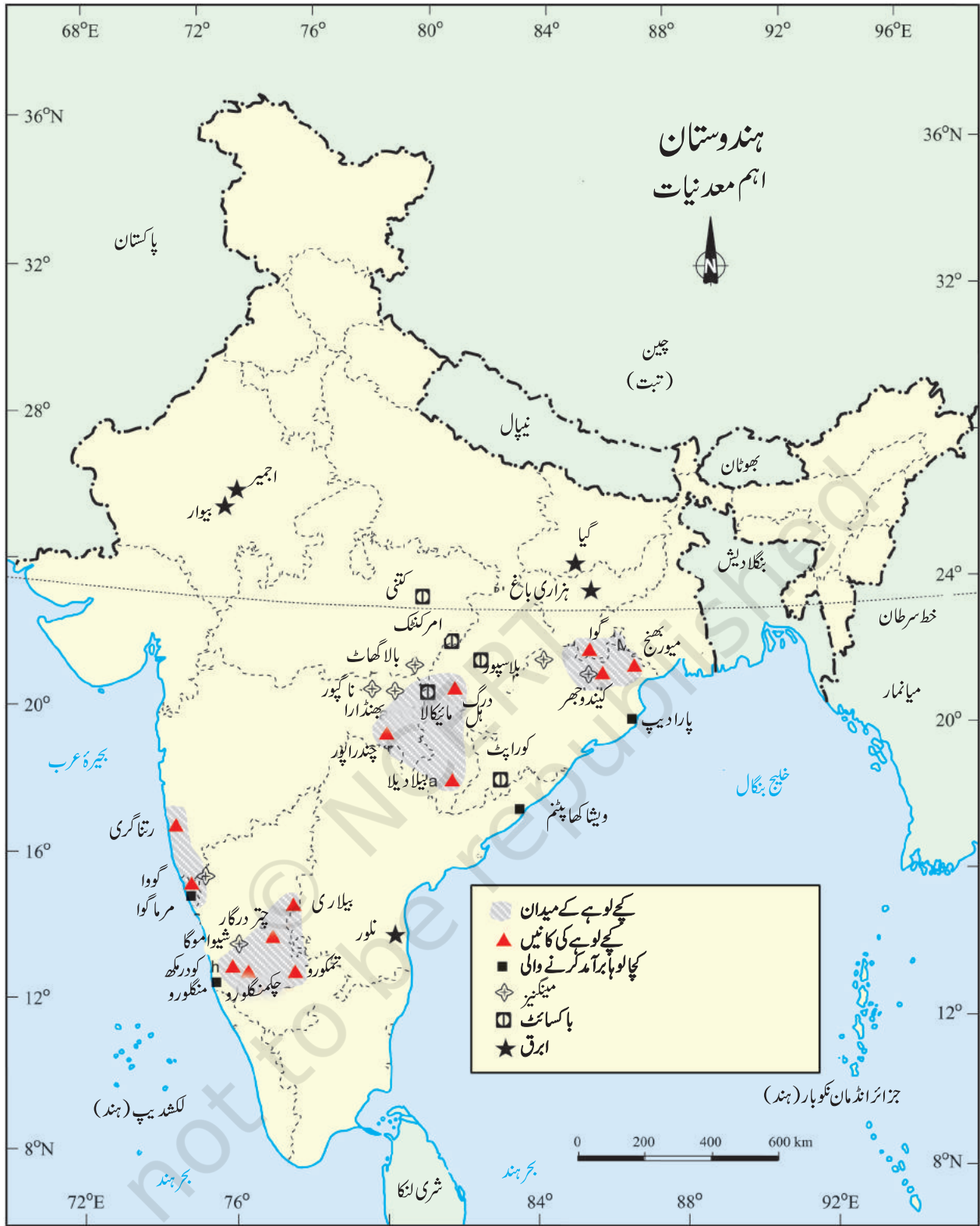
ہندوستان : کچے لوہے، مینگیز، باکسائٹ اور ابرق کی تقسیم
