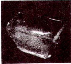
Ice( solid)
