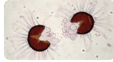
(ஆ) கிளிஸ்டோதீசியம்
