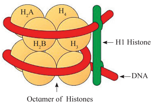
Fig. 4.5 : Nucleosome
