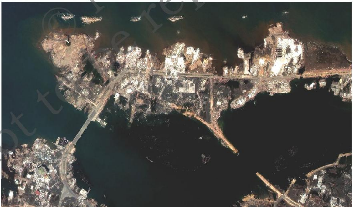
चित्र 7.10 (ख) दिसंबर 2004 में सूनामी के पश्चात् अर्जित प्रतिबिंब
