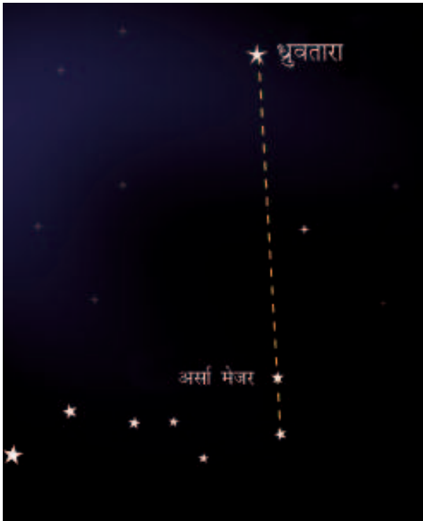
चित्र 17.13 : ध्रुव तारे की स्थिति ज्ञात करना।
