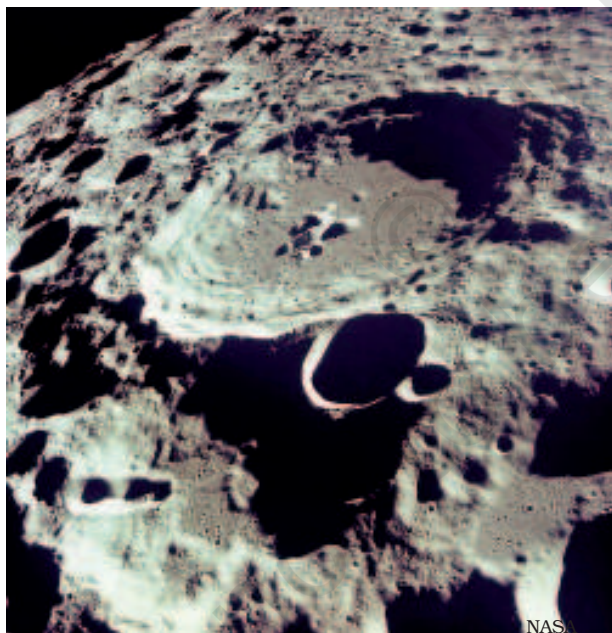
चित्र 17.7 : चन्द्रमा का पृष्ठ।
