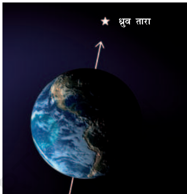
चित्र 17.10 : ध्रुव तारा पृथ्वी के घूर्णन अक्ष के निकट स्थित है।
