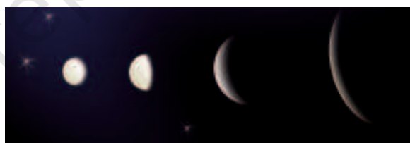
चित्र 17.20 : शुक्र की कलाएँ
