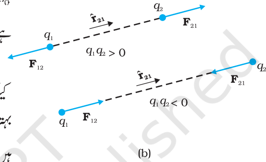
شکل 1.6 (a) جیومیٹری (b) چارجوں کے درمیان قوتیں
