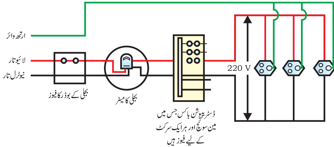
شکل 13.20 ایک عام گھریلو سرکٹ کا ڈائیگرام
