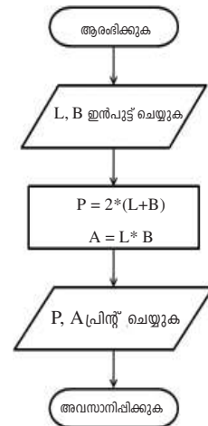
ചിത്രം 4.6 വിസ്തീർണ്ണം ചുറ്റളവ് കാണാനുള്ള ഫ്ലോചാർട്ട്
