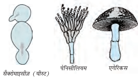
चित्र 7.3: फ़ंजाई
