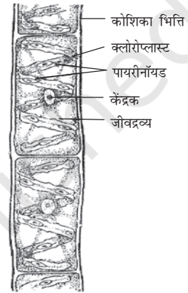
स्पाइरोगाइरा
